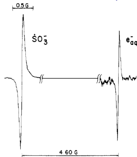
Спектр ЭПР e^-_{aq} при 296 K
